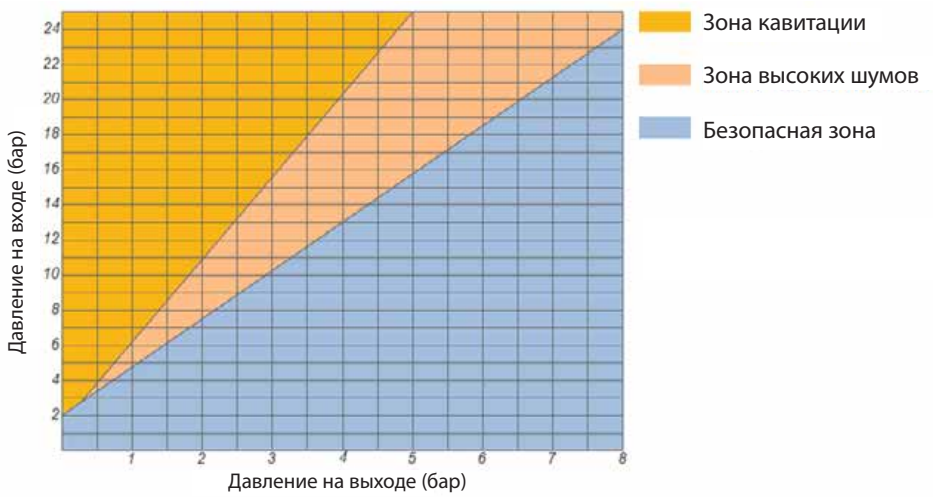
Диаграмма кавитации
