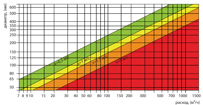
диаграмма подбора
