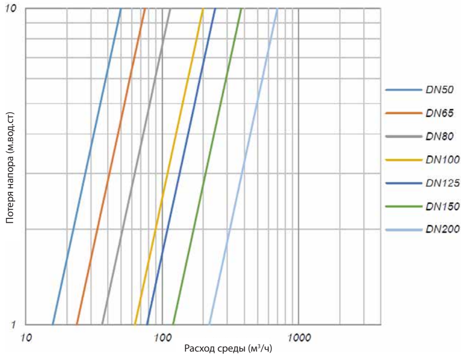
Диаграмма расхода
