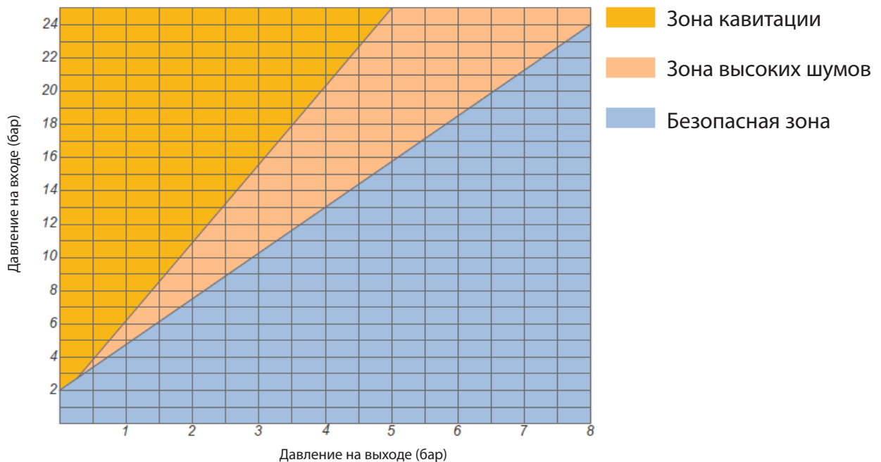
Диаграмма кавитации
