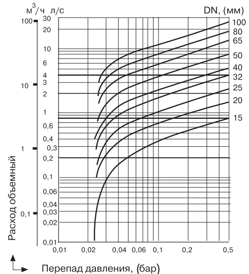
Диаграмма падения давления на клапане
